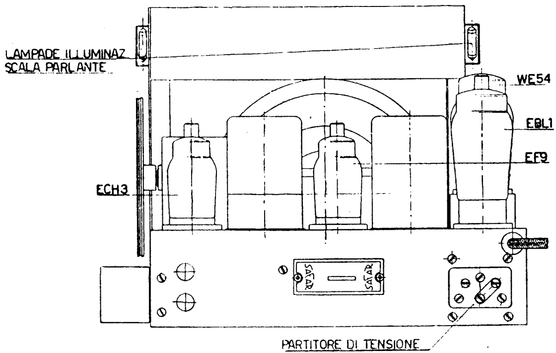
Due viste del telaio « 416 » Safar.
